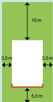
Begrenzing bouwvlak
